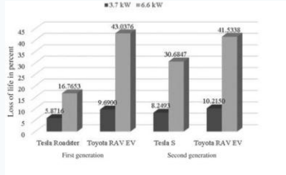
نسبة الفقد السنوية من العمر الافتراضي لمحولات التوزيع
